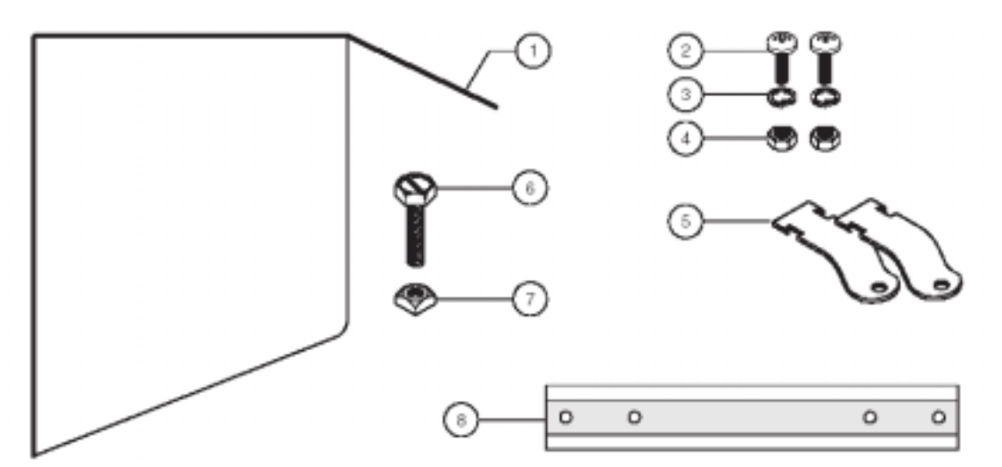
图 3-6 遮阳罩套件
